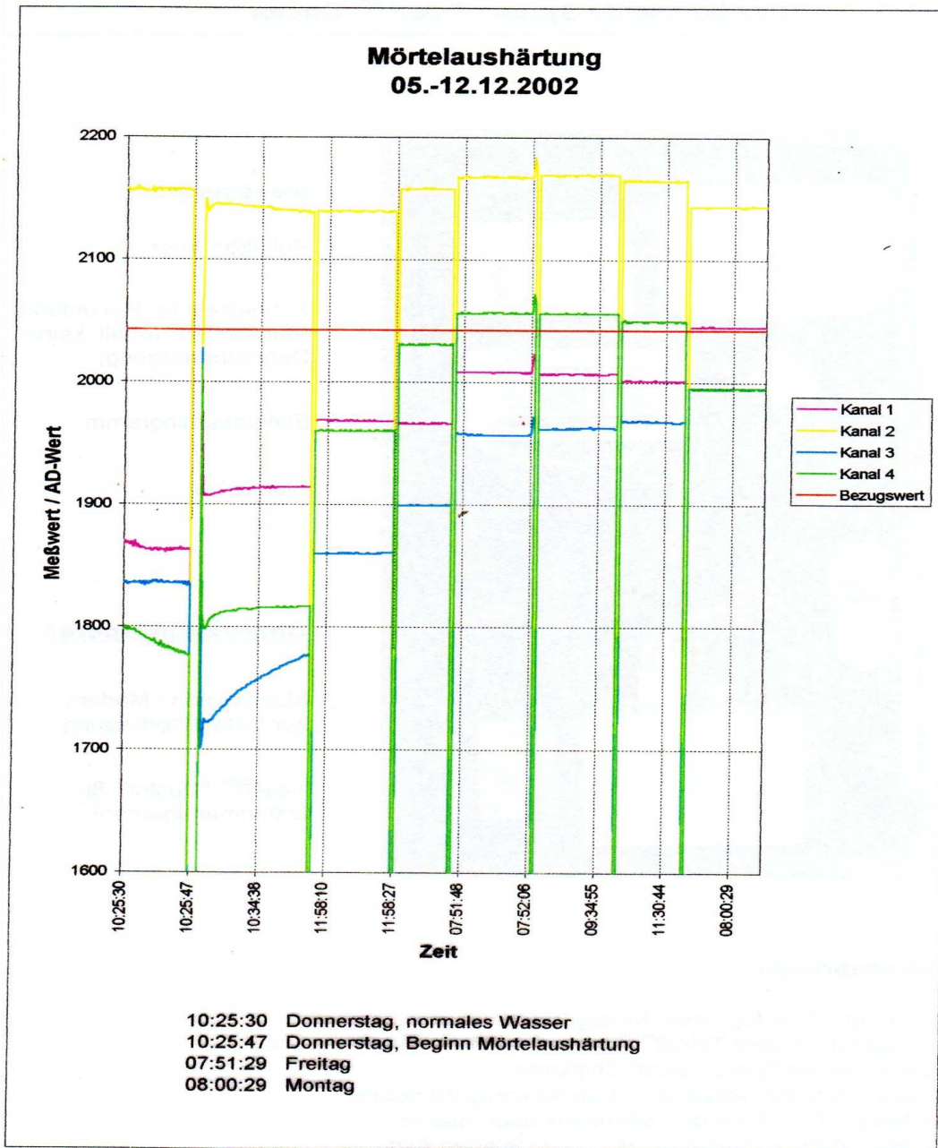
Abb. 1: Beispiel 1 für die Funktionsfähigkeit des Betonsensors
