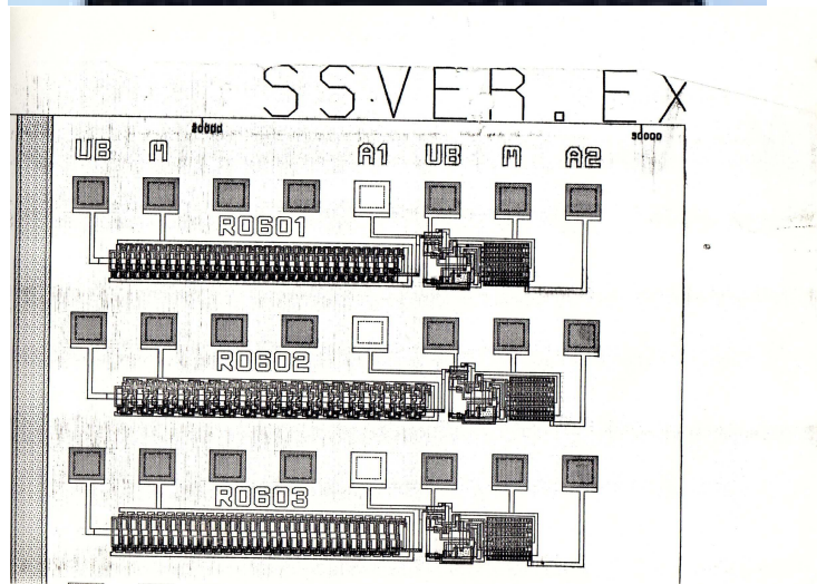
Temperatursensor mit Mikrokelvinauflösung. Frequenzanaloge Signalabgabe. Muster auf Siliziumscheibe und kontaktierte Muster.
